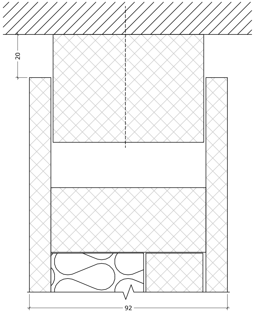
DEKO PD detail (Portal door)
