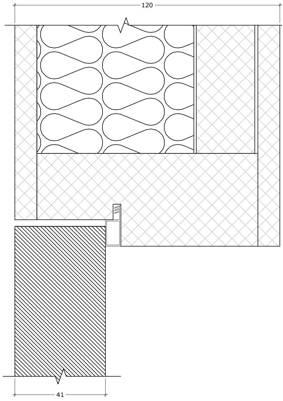
DEKO PD detail (Portal door)
