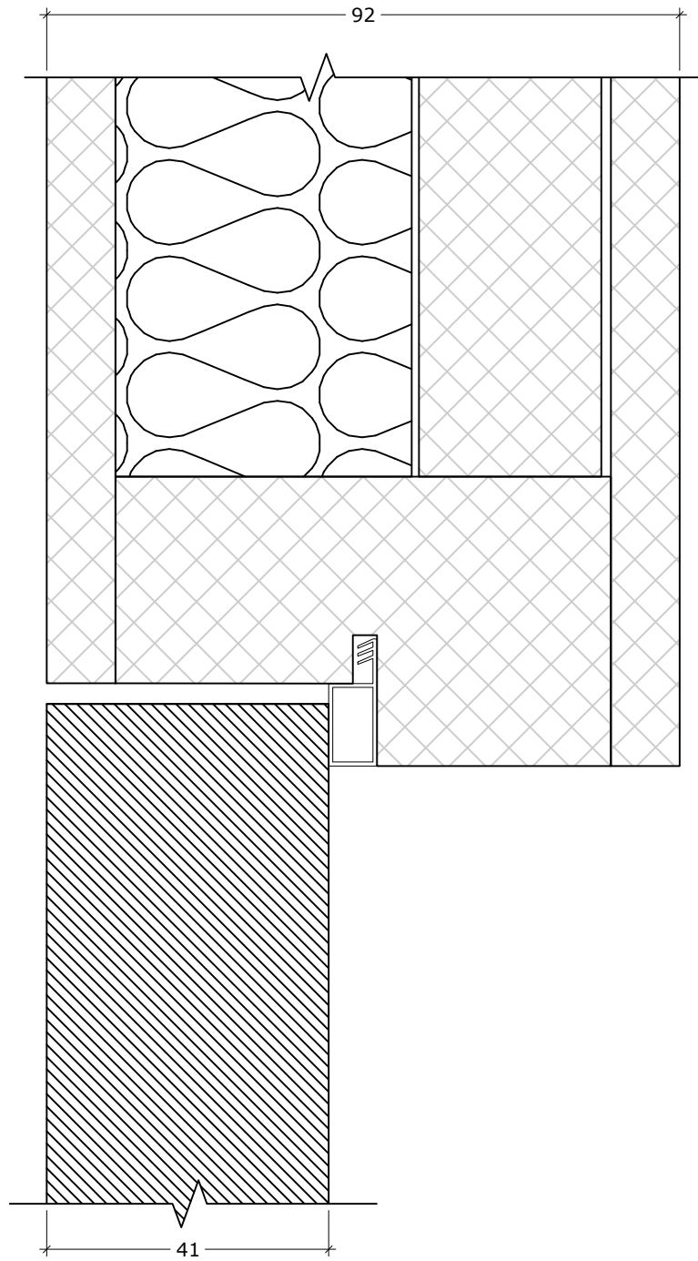
DEKO PD detail (Portal door)
