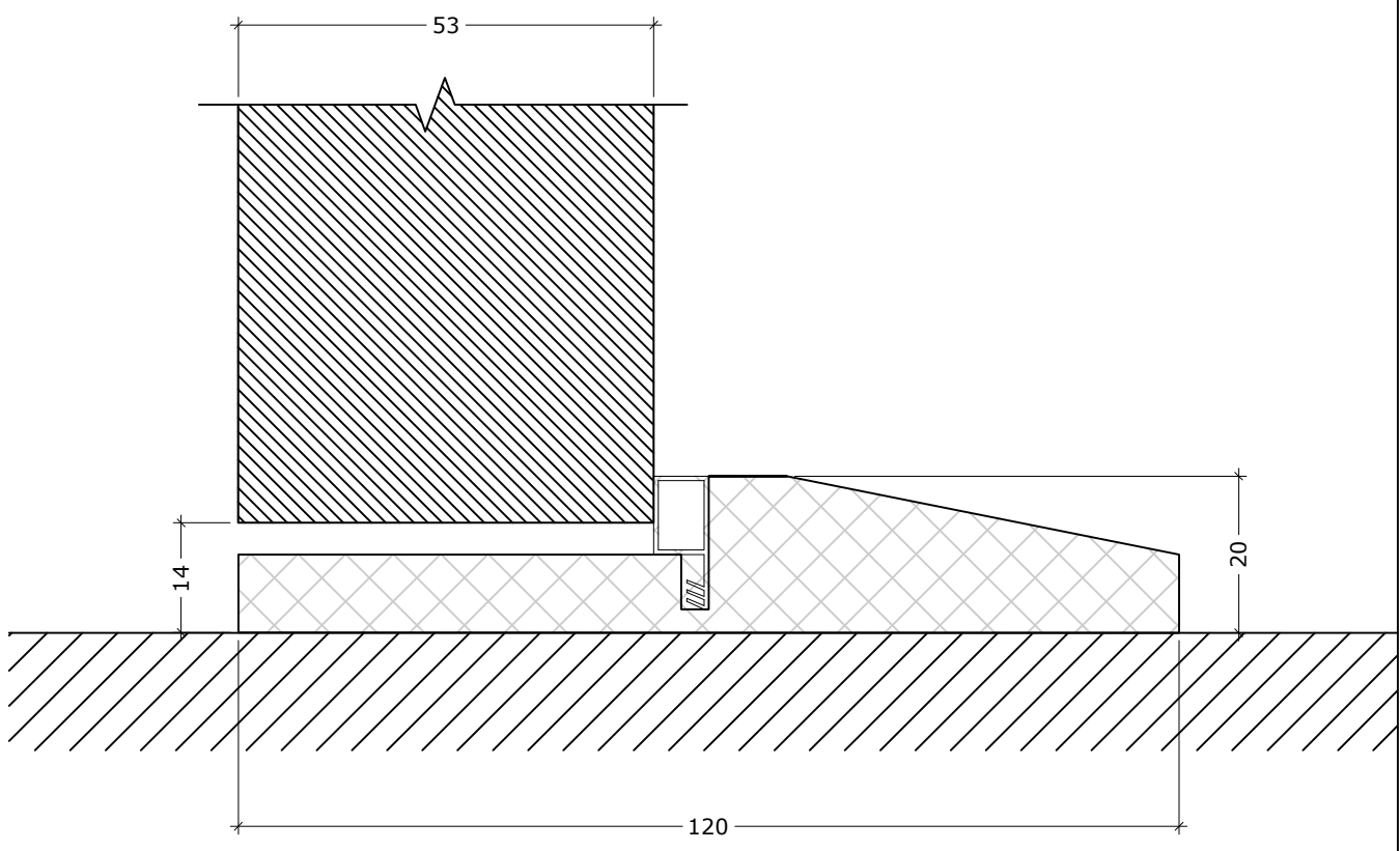
DEKO PD detail (Portal door)
