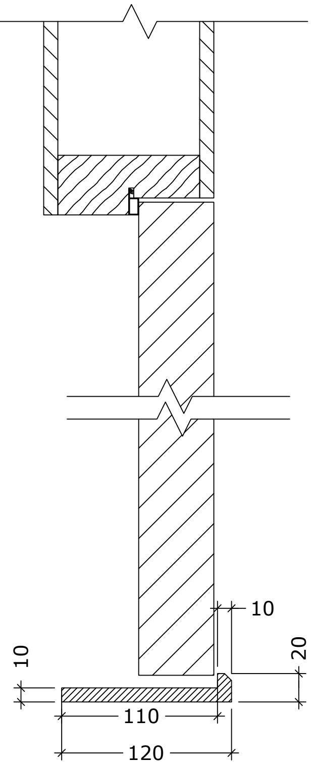
Inåtgående Portal
