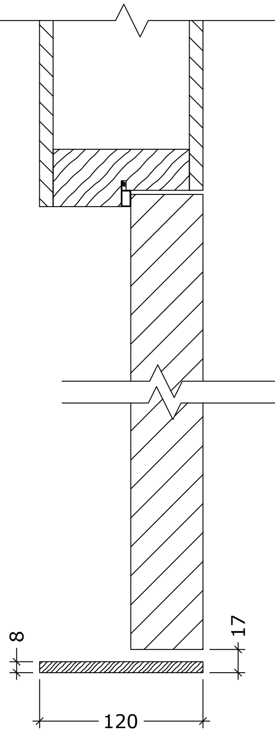
Plattröskel
