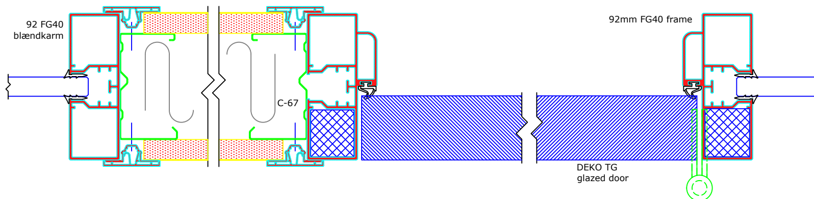
SECTION A-A
